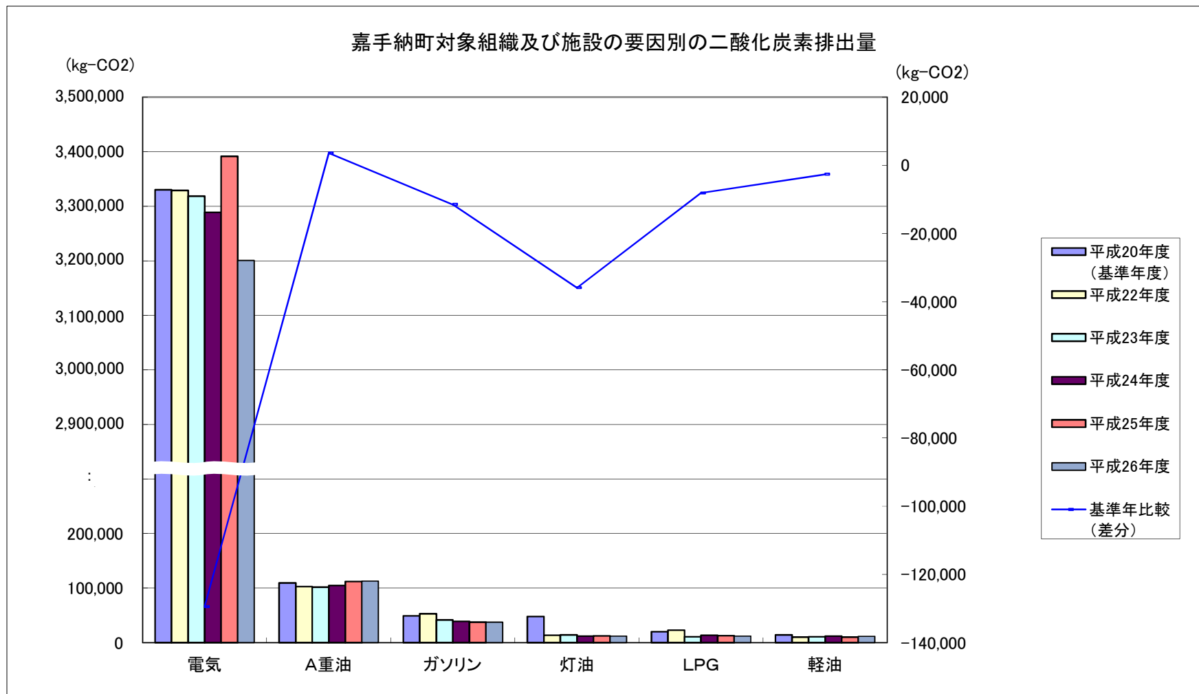
図3-2 嘉手納町対象組織及び施設の要因別の二酸化炭素排出量と経年変化 (平成22年度～平成26年)
