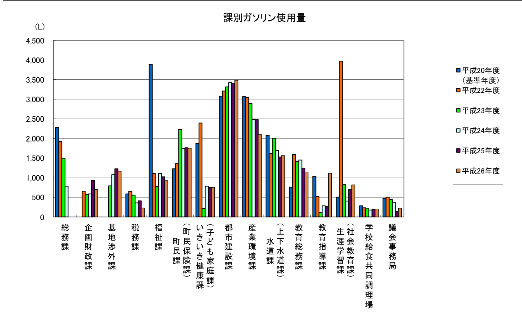
図 2-1 課別ガソリン使用量と経年変化（平成22年度～平成26年）
