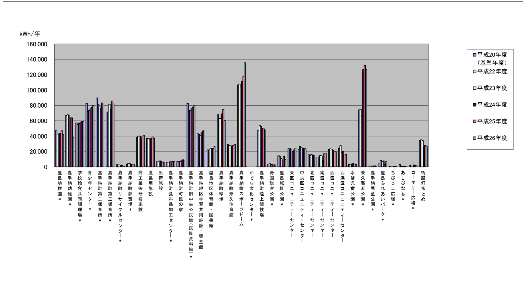
図 1-4 施設別電気使用量と経年変化(140,000kWh/年以下) (平成22年度～平成26年)
